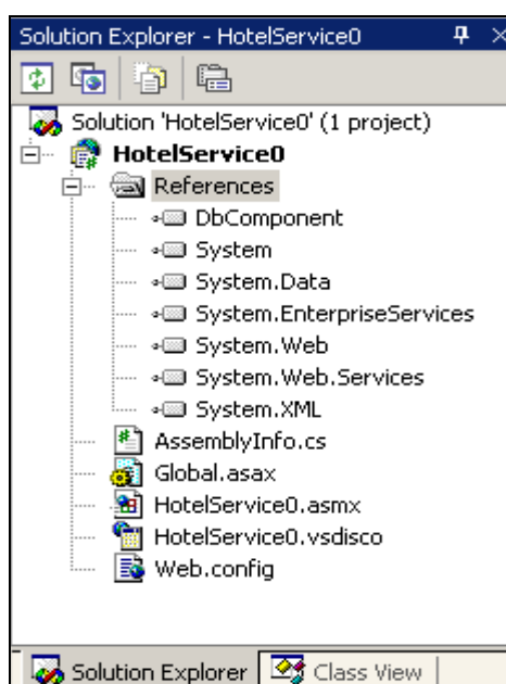
รูปที่ 2-3 หน้าต่าง Solution Explorer เมื่อทำการ Add DbComponent แล้ว
